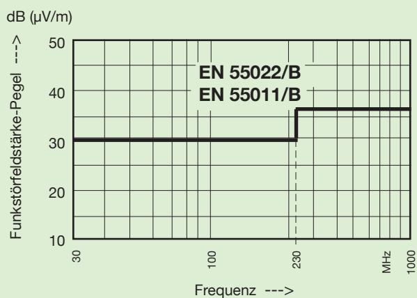
Abb. 7 Grenzwertklasse von 30MHz bis 1000MHz
