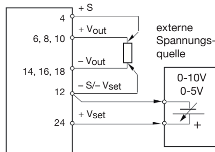
Abb. 4 Anschlussschema Spannungsprogrammierung
