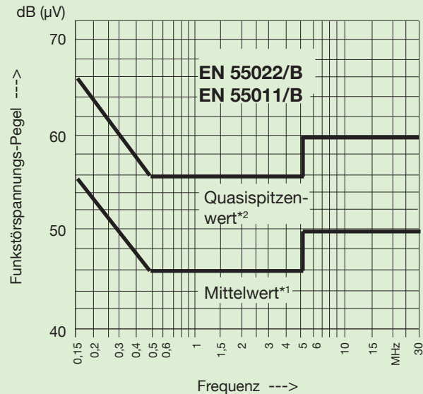
Abb. 6 Grenzwertklasse von 150KHz bis 30MHz
