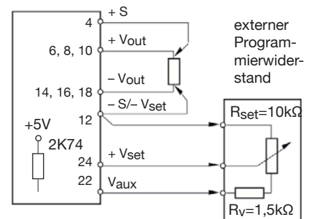
Abb. 5 Anschlussschema Widerstandsprogrammierung
