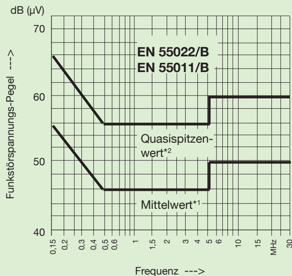
Abb. 12 Grenzwertklasse von 150KHz bis 30MHz
