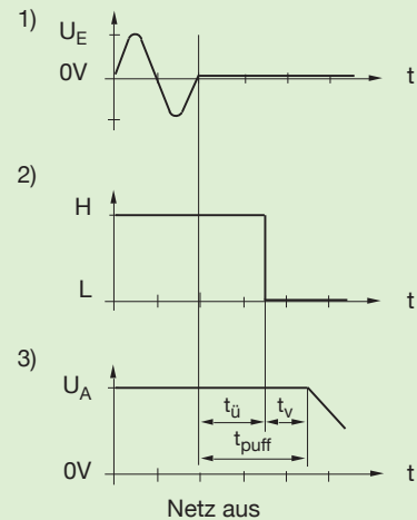
Abb. 7 Signalzuordnung PFS Low - Active
