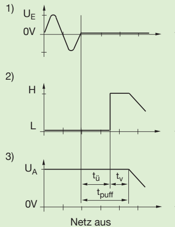
Abb. 5 Signalzuordnung PFS High - Aktiv
