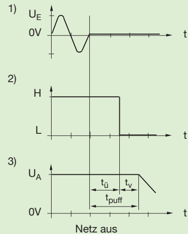
Abb. 7 Signalzuordnung PFS Low - Aktiv
