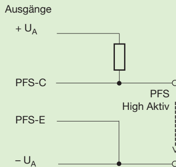
Abb. 5 Signalzuordnung PFS High - Aktiv
