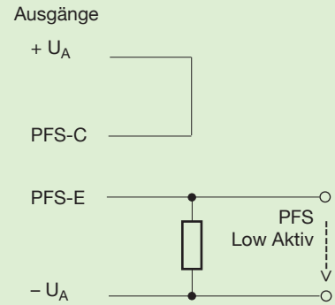
Abb. 7 Signalzuordnung PFS Low - Aktiv
